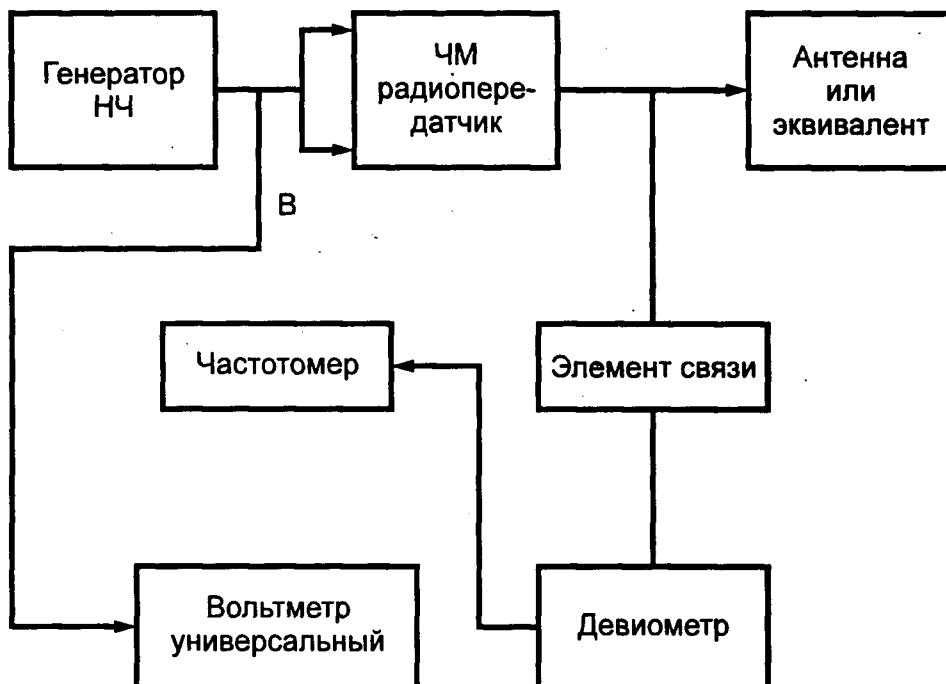
Рисунок 1 — Схема измерений параметров систем стереофонического радиовещания
